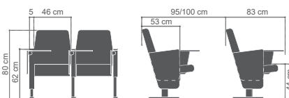
VERSIONE CON TAVOLETTA SCRITTOIO VERSION WITH WRITING TABLET
